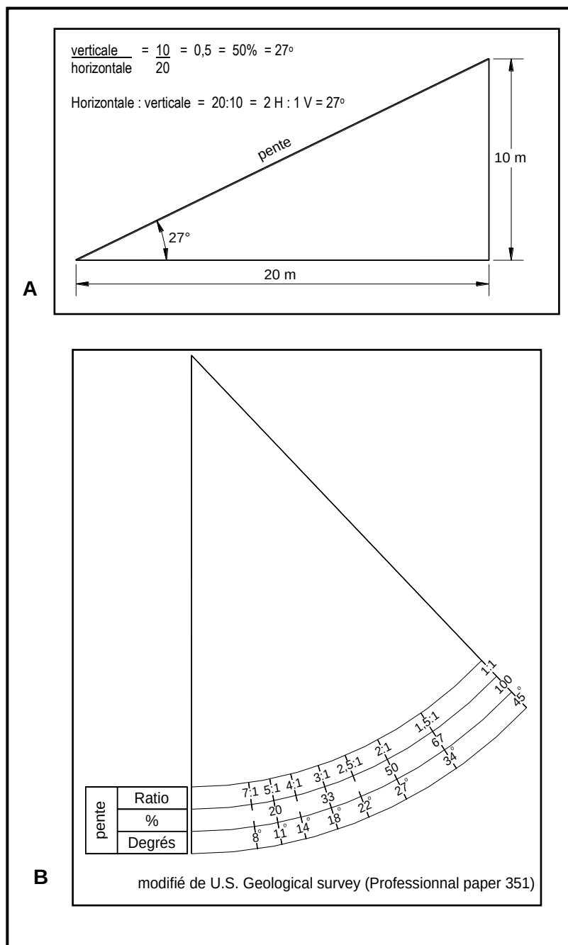
Figure 3 : Illustrations des diverses façons d'exprimer une inclinaison (A : en degré, en pourcentage et en proportion, B : correspondance entre les trois systèmes de mesure)
